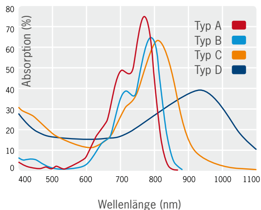
NIR-Absorber in Polycarbonat (800 bis 1100 nm)
