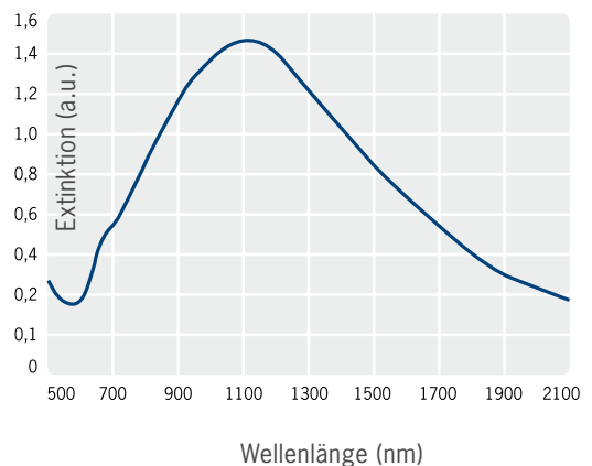
NIR-Absorber in Polycarbonat (900 bis 1500 nm)
